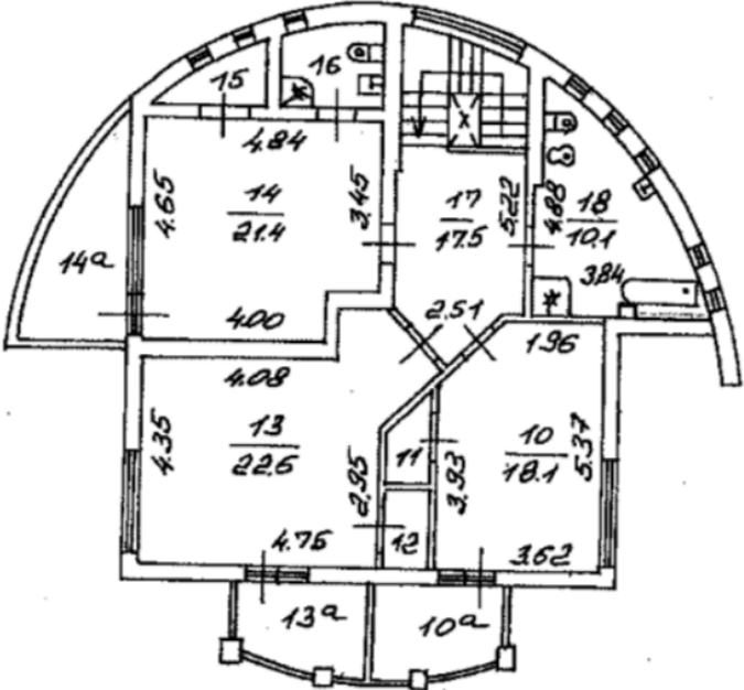
2 ЭТАЖ
