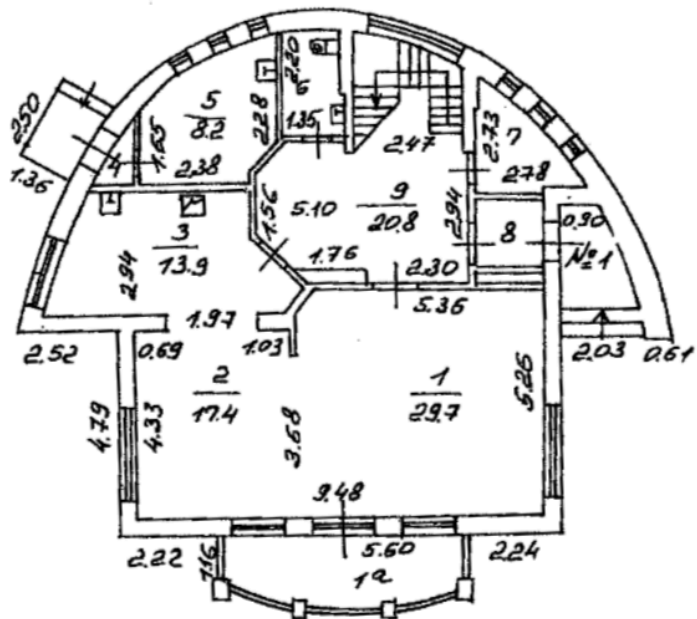
1 ЭТАЖ
