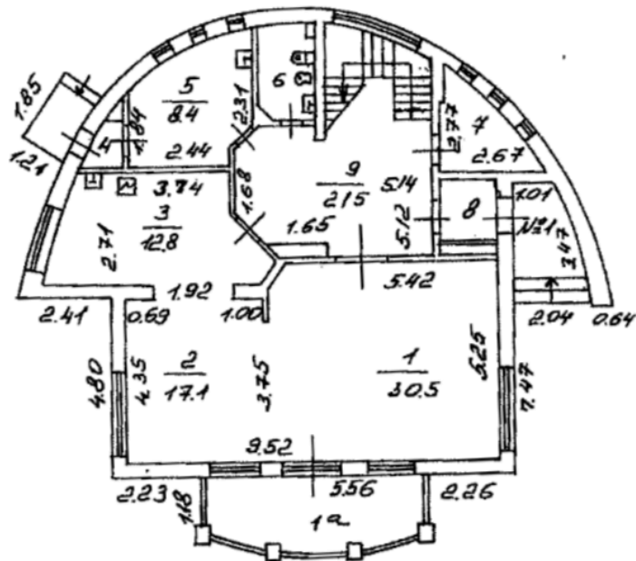
1 ЭТАЖ
