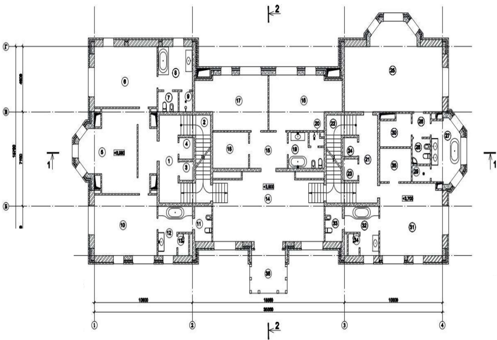
2 ЭТАЖ
