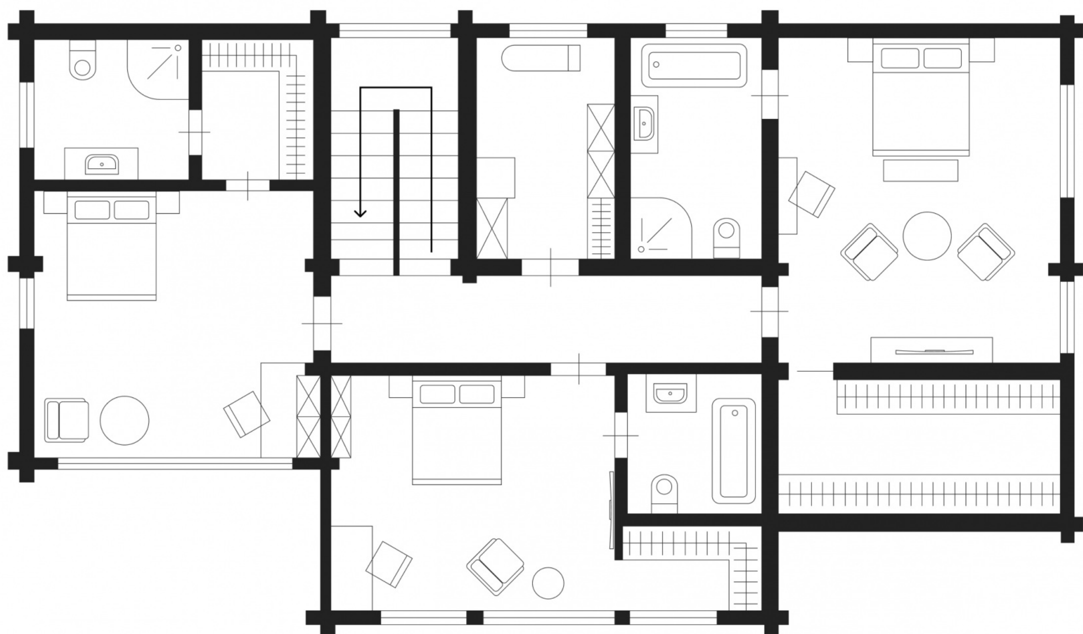
План 2-го этажа
