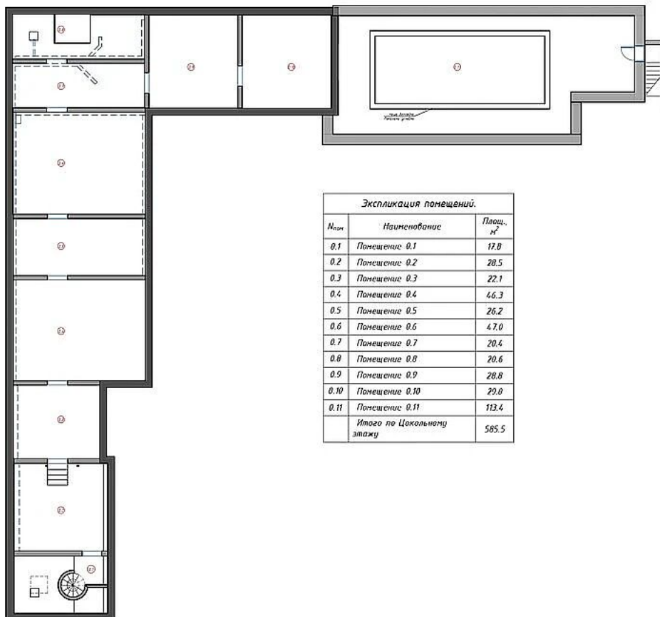
Планировочное решение. Цокольный этаж.
