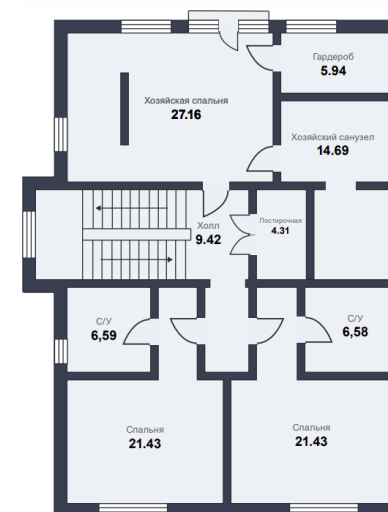
План 2 этажа
